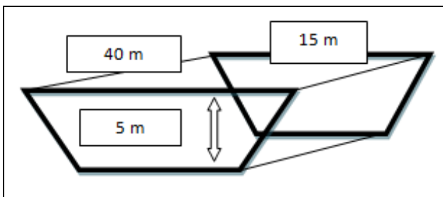
Dimensiones de la represa para los animales
