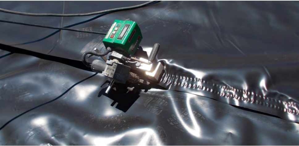
Detalle donde se muestra como la soldadora une dos paños de geomembrana.
