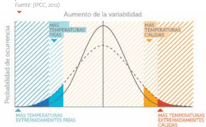
Gráfico 4: Efectos de un aumento de la variabilidad de la temperatura, achatamiento de la curva de distribución normal. Fuente: (IPCC, 2012)
