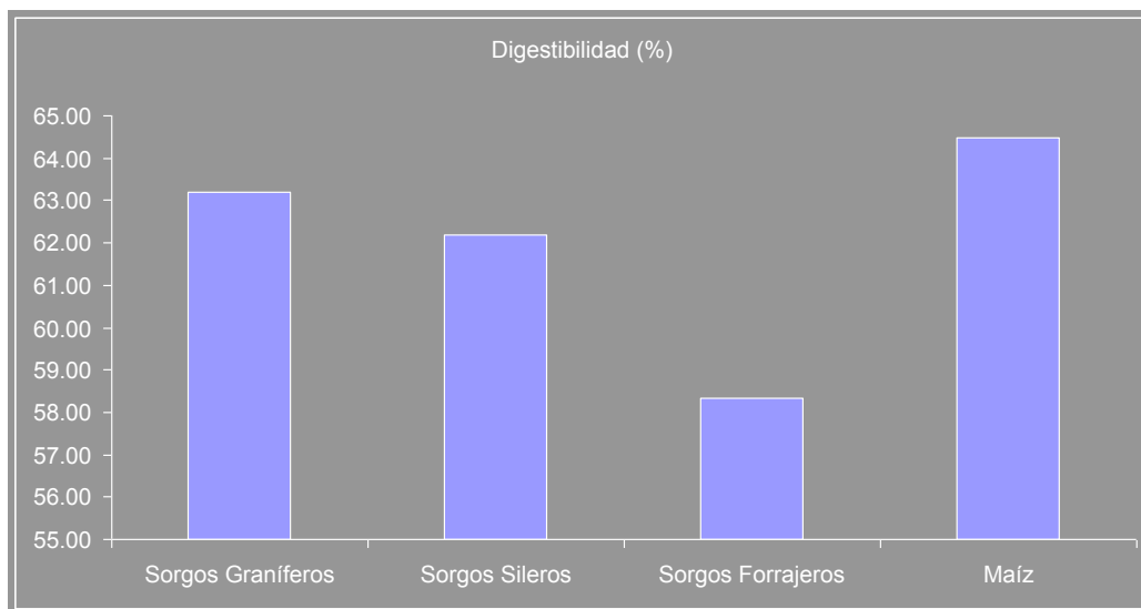
Gráfico 2: Digestibilidad promedio de silajes de distintos tipos de sorgos y maíces.
