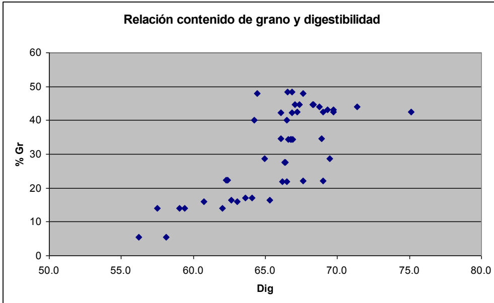
Gráfico 3. Relación entre el contenido de grano de silajes y su digestibilidad.
