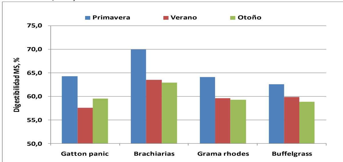
Figura 4. Digestibilidad por grupos de especies según la estación (Adaptado de Cornacchione, 2008).
