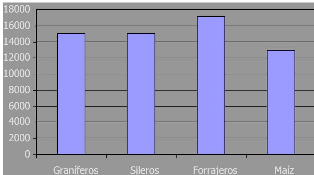
Gráfico 1: Rendimiento (Kg MS/ha) promedio de 10 años de distintos tipos de sorgos y maíces para silajes.
