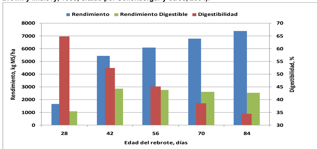
Figura 3. Efecto de la edad del rebrote sobre el rendimiento de materia seca, digestibilidad y el rendimiento de materia seca digestible de gramíneas megatérmicas (Adaptado de Brown y Mislevy, 1988; citado por Solleberger y otros, 2004).
