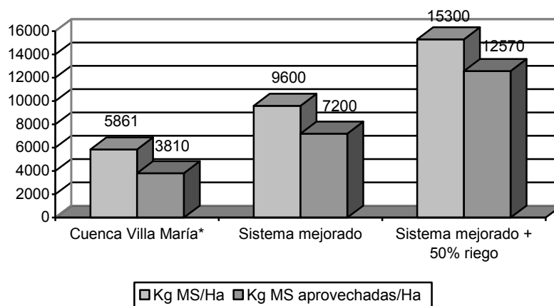
Gráfico 1. Impacto en la oferta de Kg MS/Ha
