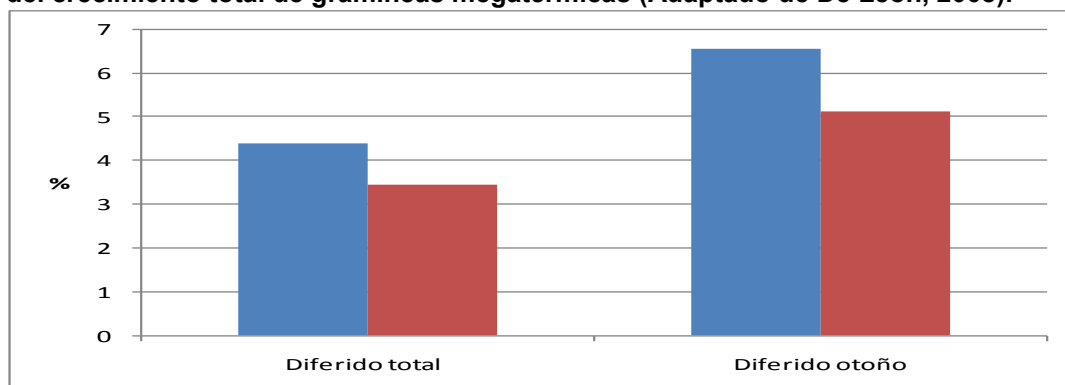
Figura 5. Contenido de proteína de la hoja y el tallo de forrajes diferidos en pie de otoño o del crecimiento total de gramíneas megatérmicas (Adaptado de De León, 2008).
