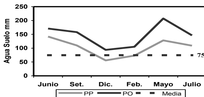
Figura 3: Variación del agua disponible en el perfil del suelo (mm/80 cm) bajo pastura polifítica y pasto ovillo. 75 mm representa el punto de marchitez permanente.
