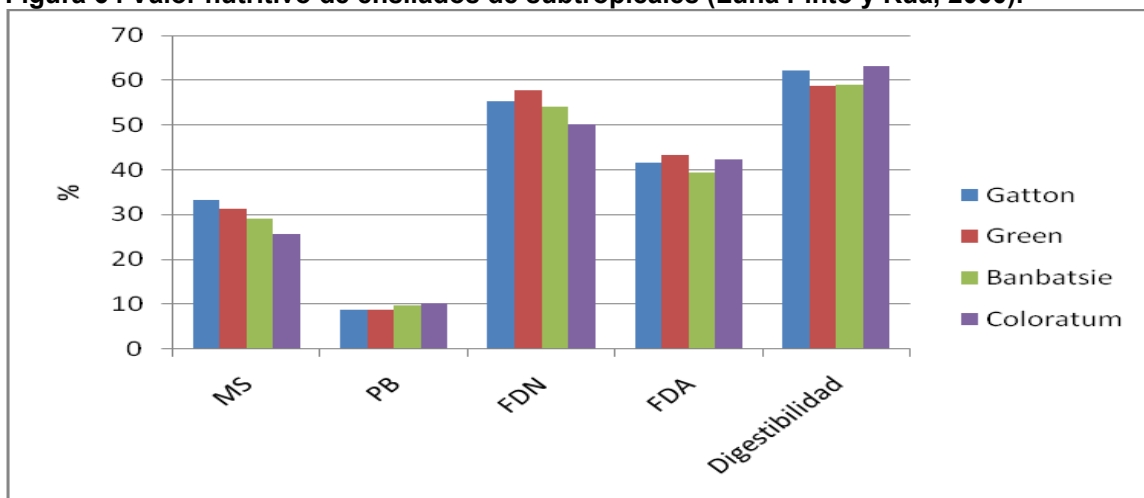
Figura 6 . Valor nutritivo de ensilados de subtropicales (Luna Pinto y Rua, 2000).
