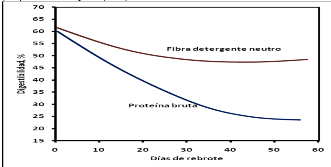
Figura 3. Efecto de la edad del rebrote sobre el rendimiento de materia seca, digestibilidad y el rendimiento de materia seca digestible de gramíneas megatérmicas (Adaptado de Brown y Mislevy, 1988; citado por Solleberger y otros, 2004).
