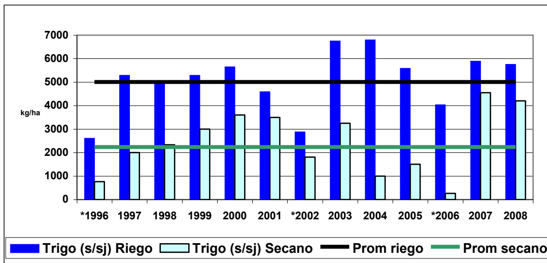
Rendimientos de Trigo (kg/ha) en riego y secoano
