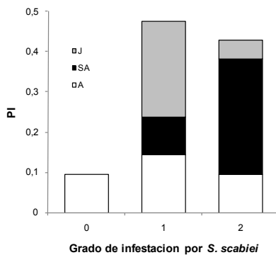
Fig. 1. Estructura etaria y proporción de individuos (PI) pertenecientes a los diferentes grados de infestación por Sarcoptes scabiei detectados en carpinchos en dos humedales artificiales (tajamares) de los Esteros del Iberá, Corrientes, Argentina. A: adultos; SA: subadultos; J: juveniles; 0: sin carga parasitaria evidente; 1: baja carga; 2: carga elevada.
