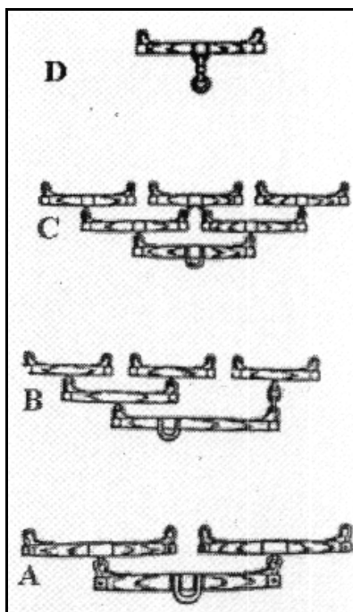
Balancines: A) Balancines de delanteros para un tiro de cuatro; B) Juego de cinco balancines para des delanteros a lo par, C) Ídem anterior, con seis balancines, B) Balancín del delantero para el unicorn (uniconio).
