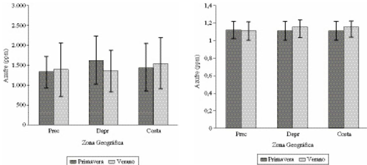
Figura 1. Concentraciones promedio (ppm) de azufre en pradera (A) y agua (B) según zona geográfica (costa: Costa, depresión intermedia: Depr y precordillera: Prec) en 45 predios bovinos de carne en los periodos de primavera 2008 y verano 2009. Cada barra de error está construida utilizando \pm 1 desviación estándar del promedio.
