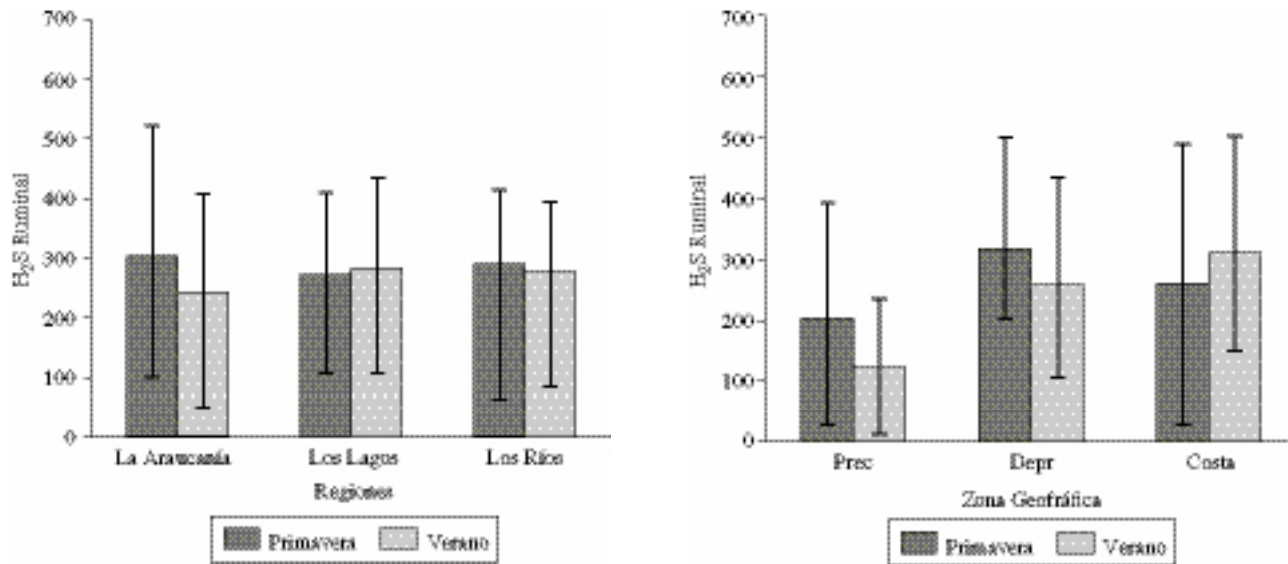
Figura 2. Concentraciones promedio (ppm) de H 2 S en gas ruminal obtenidas de 225 bovinos durante la época de primavera y verano en las regiones de La Araucanía, Los Ríos y Los Lagos de Chile (A) y en tres áreas geográficas (costa: Costa, depresión intermedia: Depr, precordillera: Prec) de cada región (B). En cada región se analizaron 75 animales. Cada barra de error está construida utilizando \pm 1 desviación estándar del promedio.
