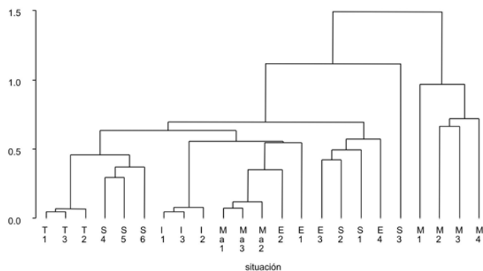
Figura 2. Dendrograma del análisis de clusters del espesor 0-100 cm bajo diferentes situaciones pertenecientes a un feedlot .
