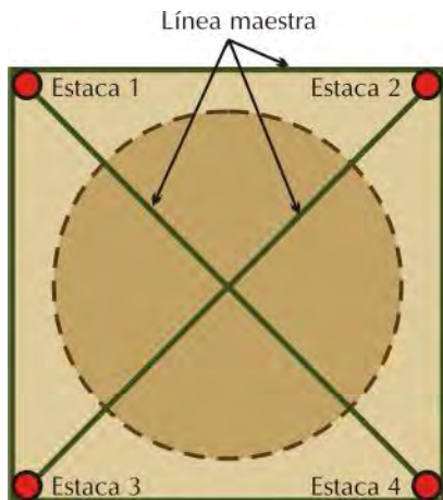
Figura 5. Esquema del trazado y postura de lienzo a través de las estacas para la nivelación del terreno.
