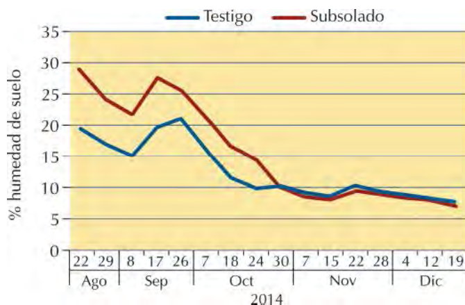
Figura 9. Humedad de suelo (%), medida a los 20 cm de profundidad, en el período agosto-diciembre de 2014. Ensayo de subsolado en fajas, en una pradera sembrada de Falaris. INIA-Hidango.
